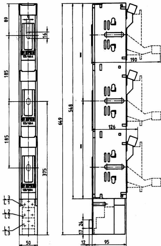
NH-pojistkový lištový odpínač, velikost 00/185: 160 A
