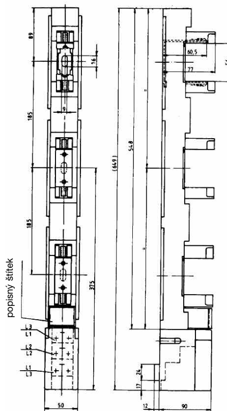
NH-pojistkové lišty velikost 00/185
