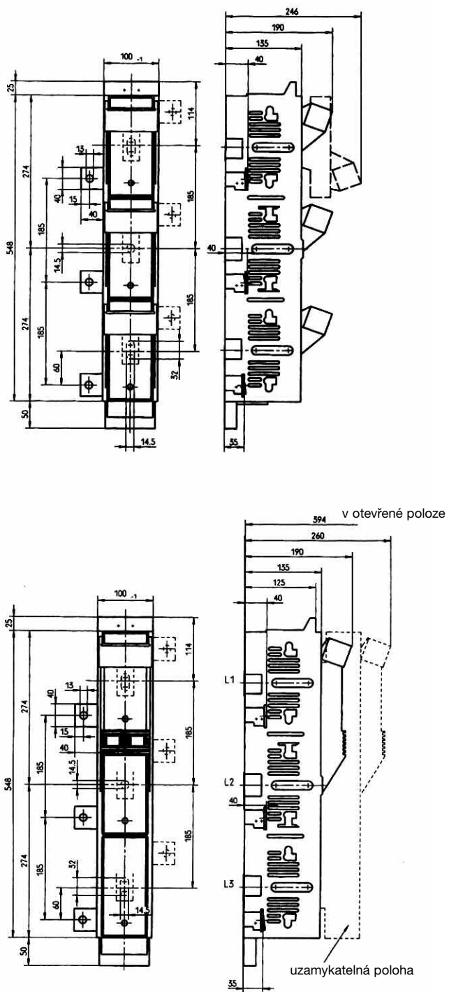
NH-pojistkové lištové odpínače řada 2000 s bočním připojením, velikost 2 - 3: 400 A - 630 A
