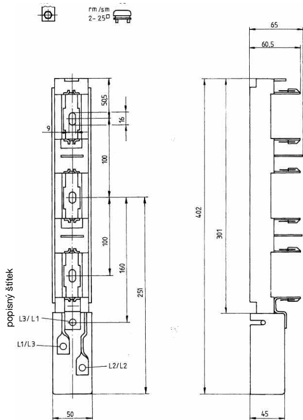
NH-pojistkové lišty velikost 00/100: 125/160 A
