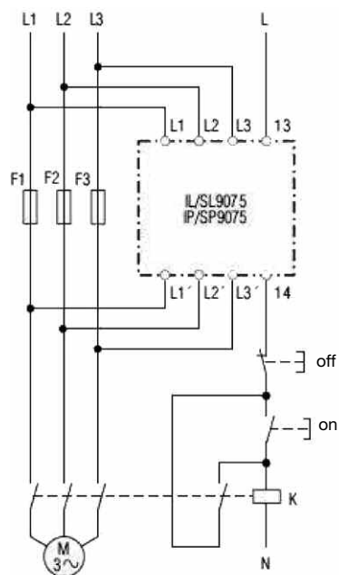
Kontrola stavu pojistek v 3-fázové síti
