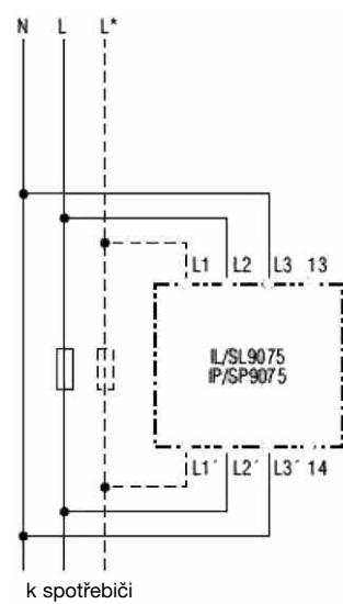
Kontrola stavu pojistek v střídavé elektrické síti
