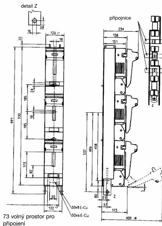
NH-pojistkové lištové odpínače, velikost 4a: 1250/1600 A
