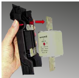
Bezdotykové odblokování NH-pojistek
