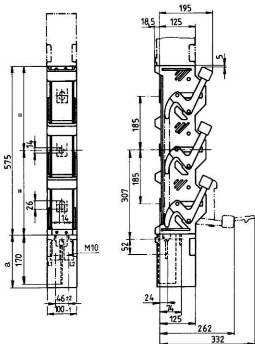
NH-pojistkové lištové odpínače, velikost 1: 250 A
