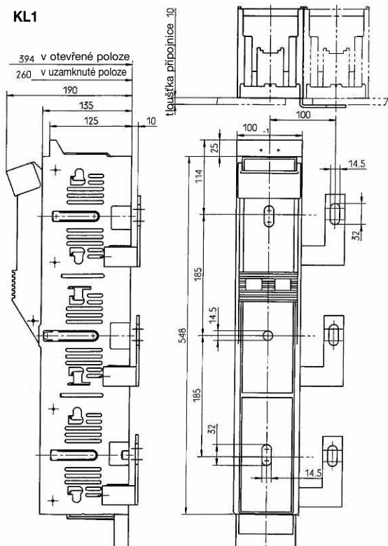
NH-pojistkové lištové odpínače, velikost 3, 3-pólové ovládání k připojení dvou systémů přípojnic
