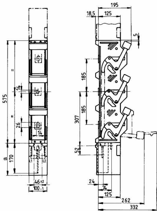
NH-pojistkové lištové odpínače, velikost 2: 400 A
