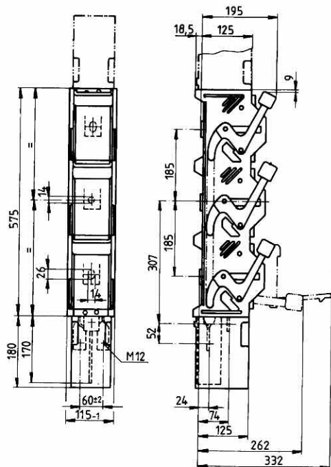
NH-pojistkové lištové odpínače, velikost 3: 630 A
