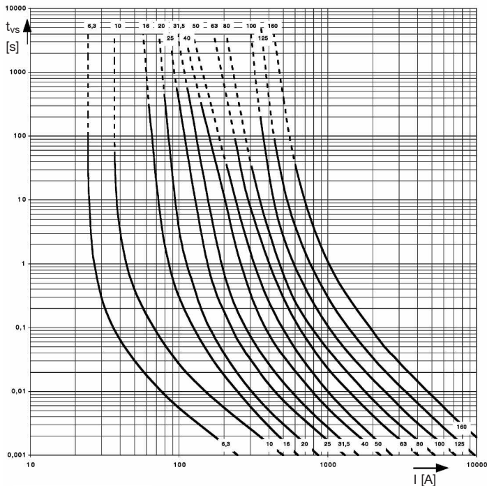
Fig.10 3/7,2 kV
